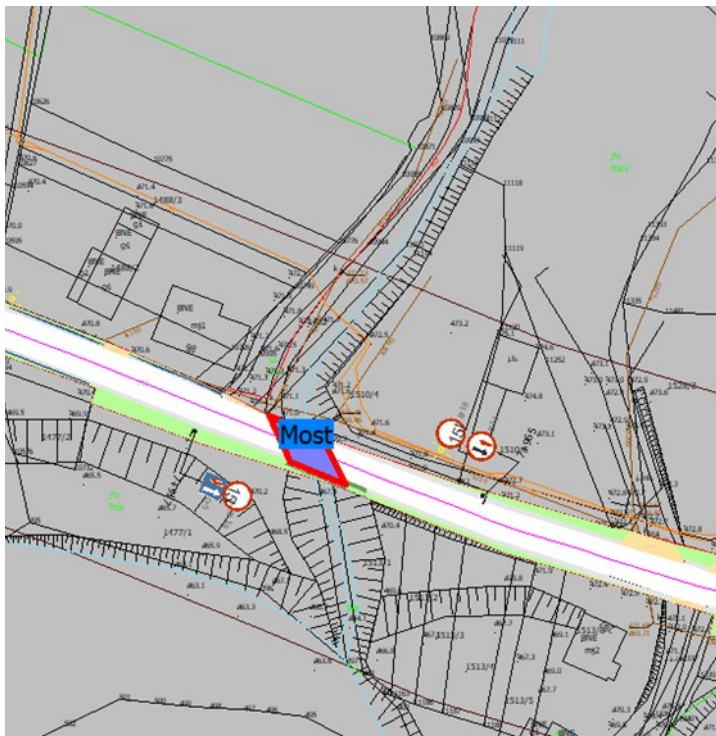
Ilustracja 3: Obiekt mostowy w ciągu DP 1425S w km 7+391 w Juszczyńce - orientacja
