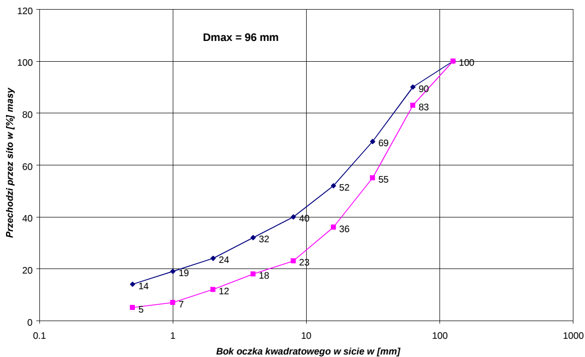
Rys. 2-4. Zalecane graniczne krzywe uziarnienia kruszywa o maksymalnej wielkości ziarn do 96 mm Tablica 2-3
